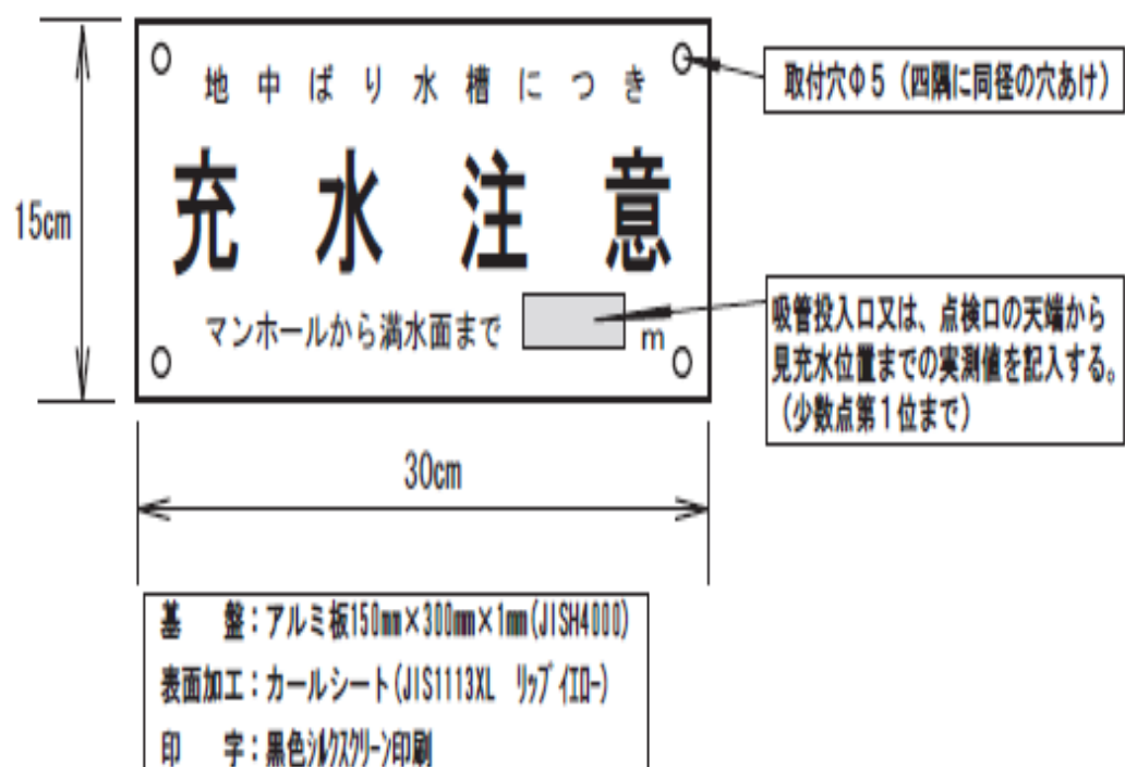
別図11 地中ばり水槽表示
