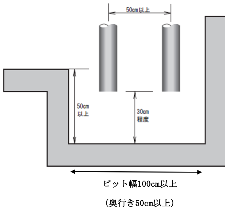
別 図 14 吸水口が集水ピット内に入る場合の設置例
