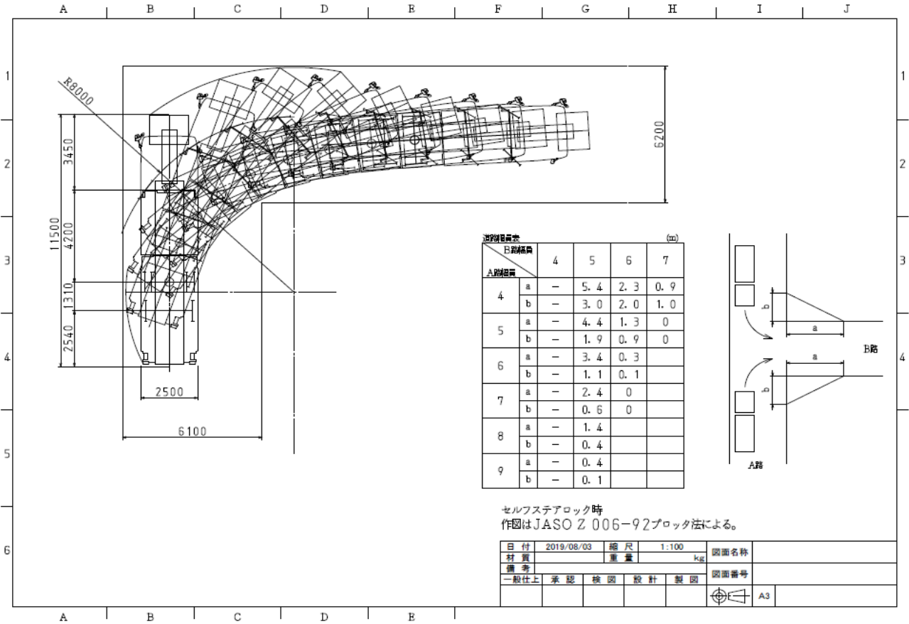
別図4 消防はしご車回転図
