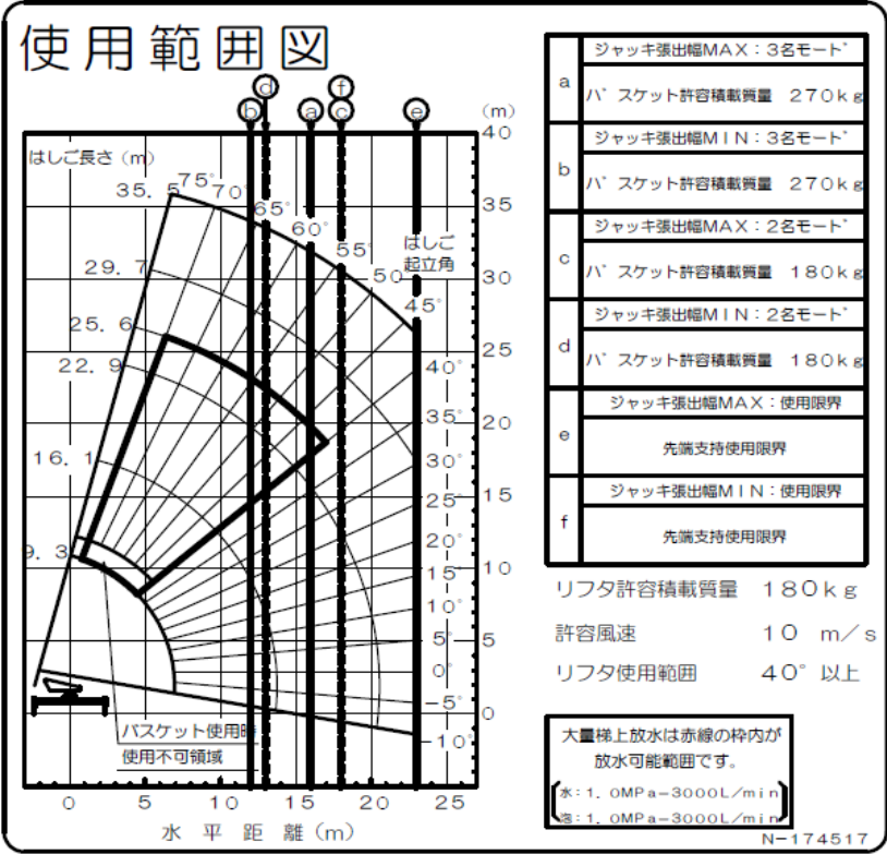
MLF5-35使用範囲図
