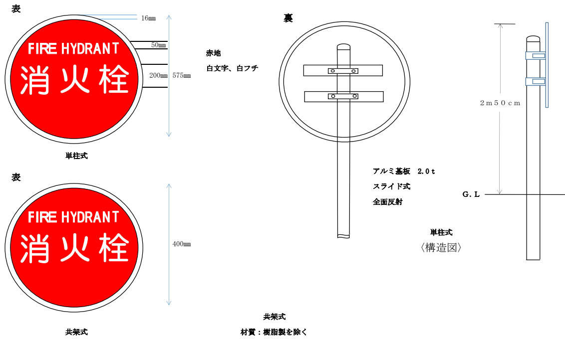
別図2 (第8条及び第13条関係) 防火水槽標識 (現場打ち鉄筋コンクリート水槽、二次製品水槽、地中ばり水槽)
