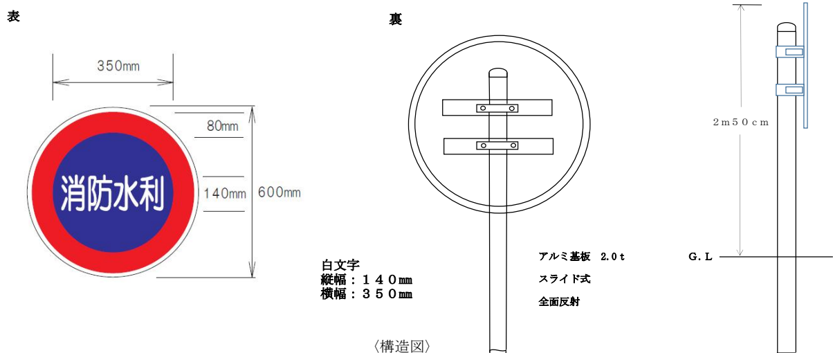
別図3 (第8条及び第13条関係) 消防水利標識 (プール等)
