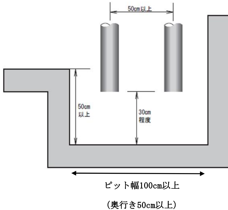
別図 1 5 (第 1 3 条関係) 吸水口が集中ピット内に入る場合の設置例
