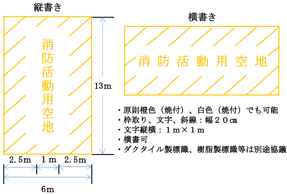
別図7 (第13条関係) 消防活動空地標識
