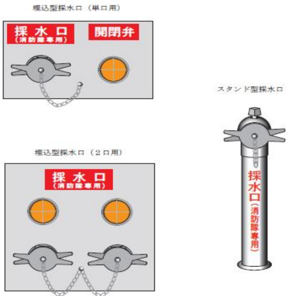
別図9 (第13条関係) 採水口 (開閉弁付)
