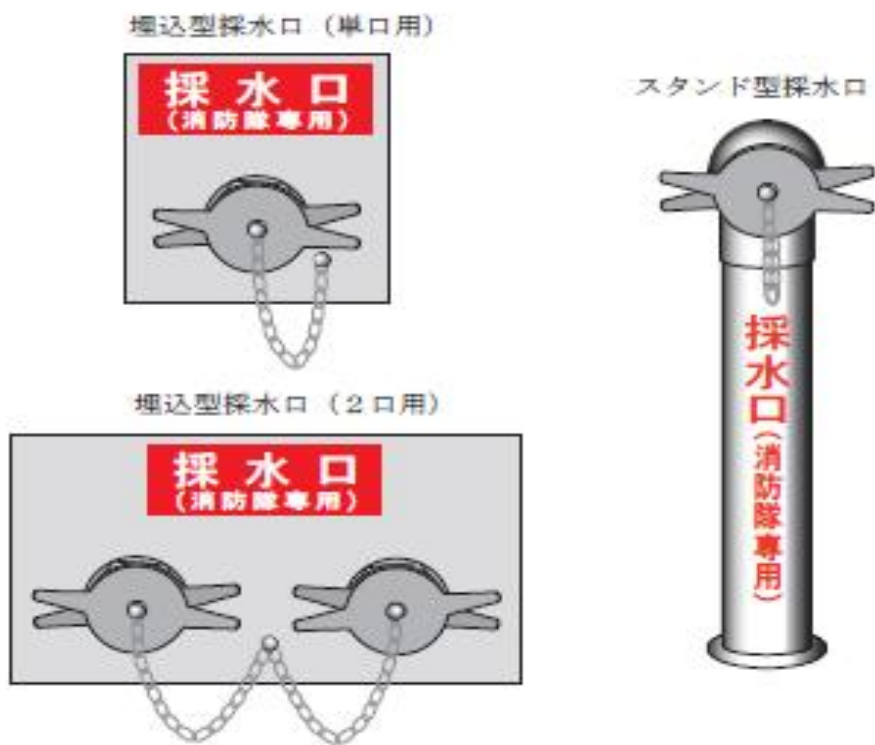
別図8 (第13条関係) 採水口
